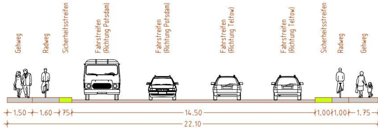
Planung (westlicher Ortseingang bis Schleusenweg)
