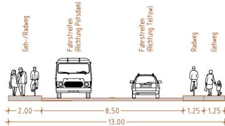
Planung (Schleusenweg bis Bauende)
