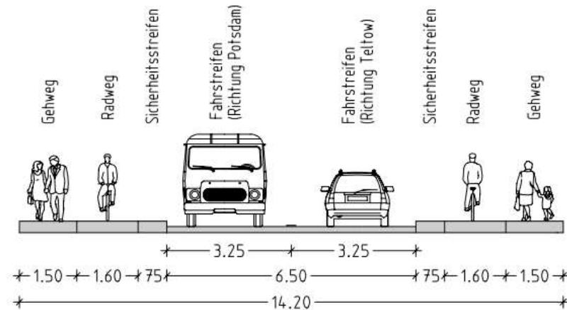
Planung (Schleusenweg bis Bauende)
