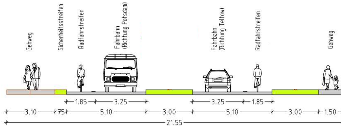
Planung (westlicher Ortseingang bis Schleusenweg)
